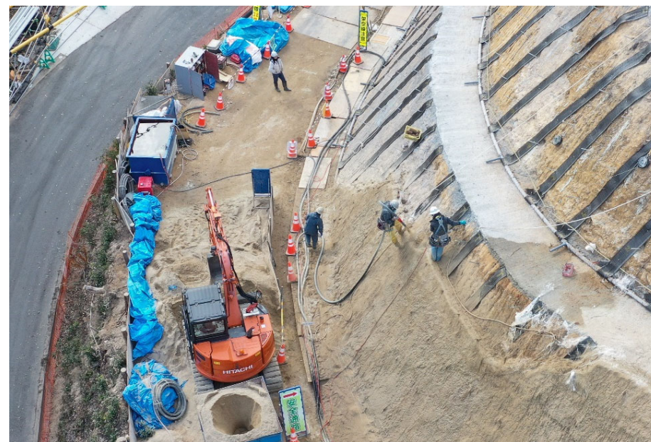
【法面工 施工状況】
