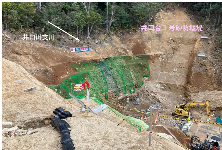
【 右岸側より 】
