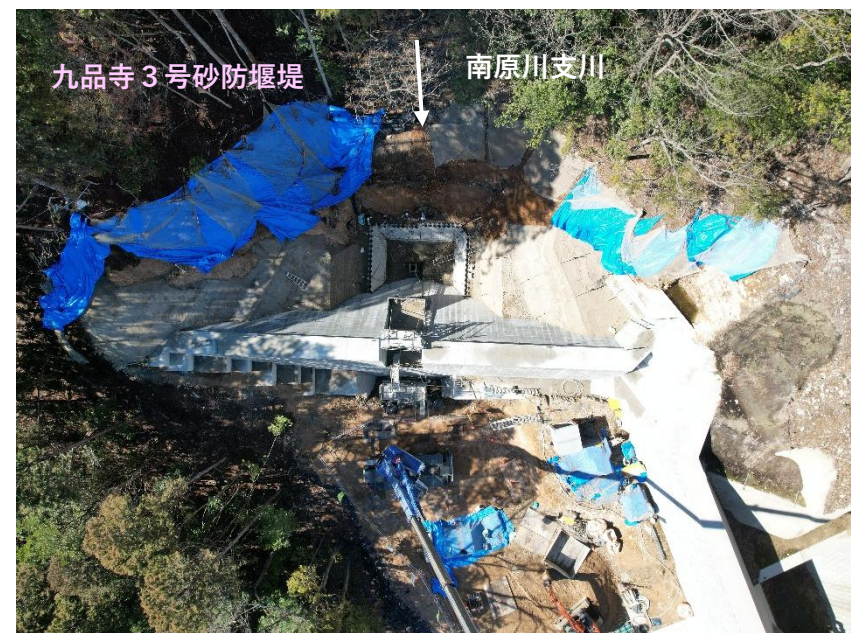
【砂防堰堤 堰堤上流側施工状況】
