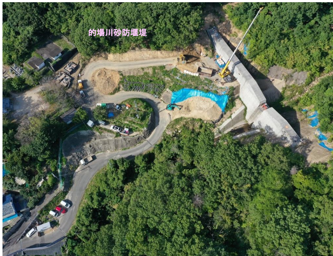
砂防堰堤全景（下流側より）
