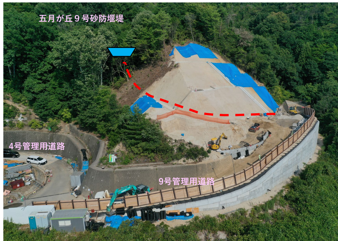
【五月が丘4、9号砂防堰堤管理道 施工状況】
