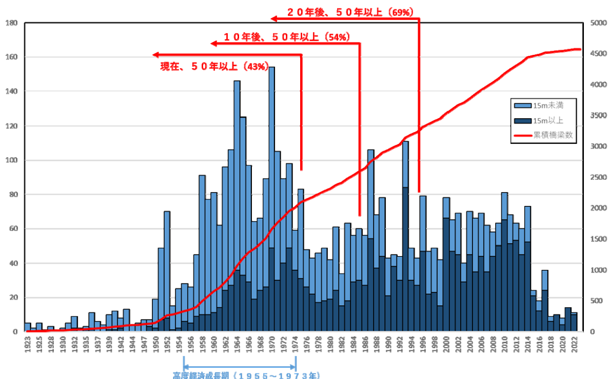
建設年次別の橋梁箇所数分布
