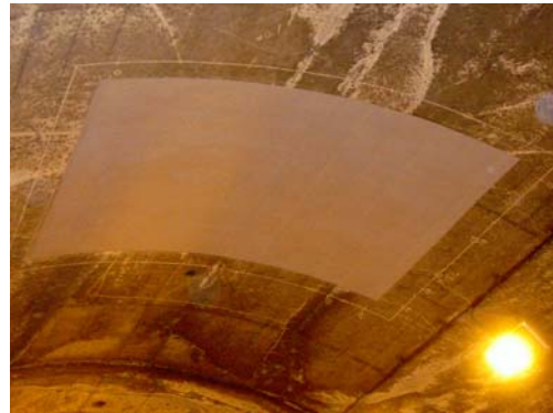
コンクリート剥落防止対策後
