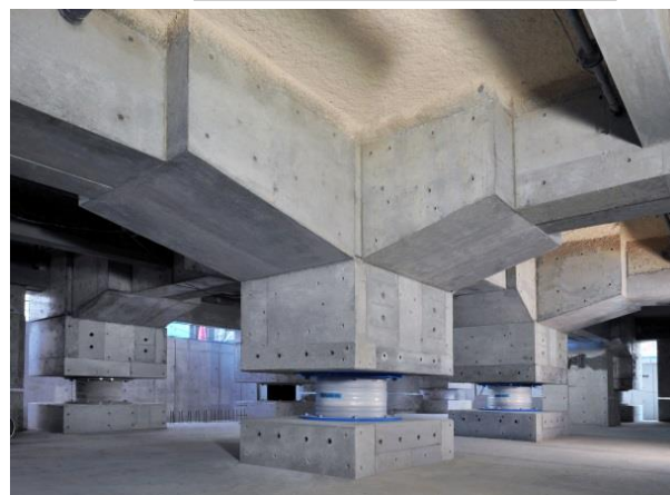
広島合同庁舎1号館の免震装置
