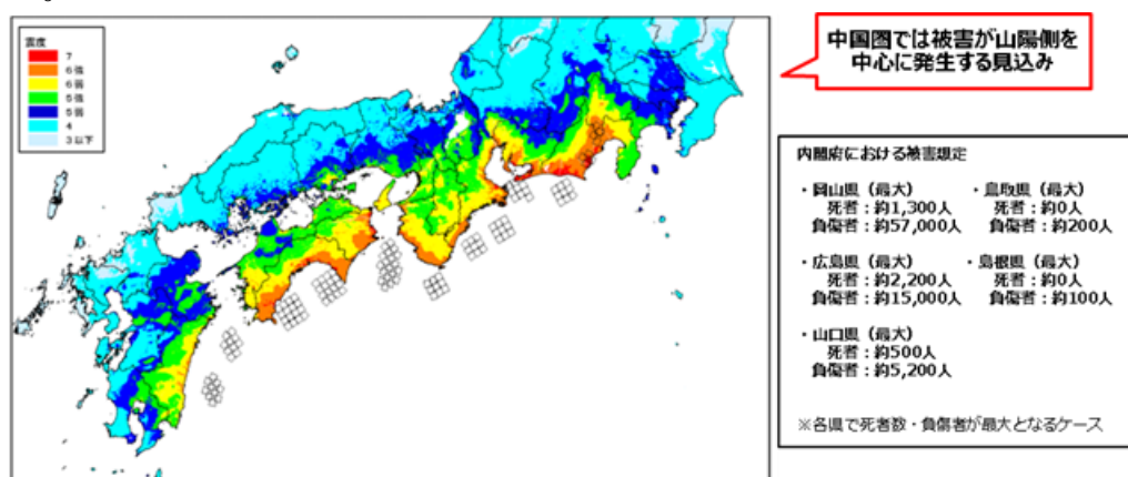
図 18 南海トラフ地震の震度分布
