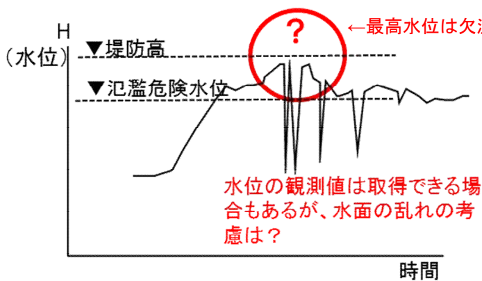
水位観測例
