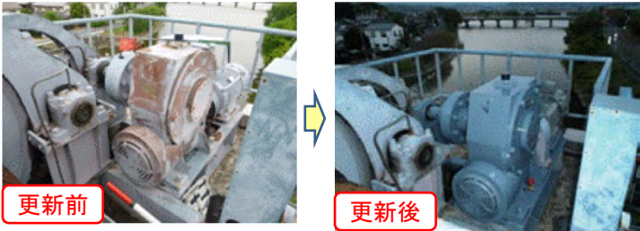
防潮水門の巻き上げ機の更新(岡山県)
