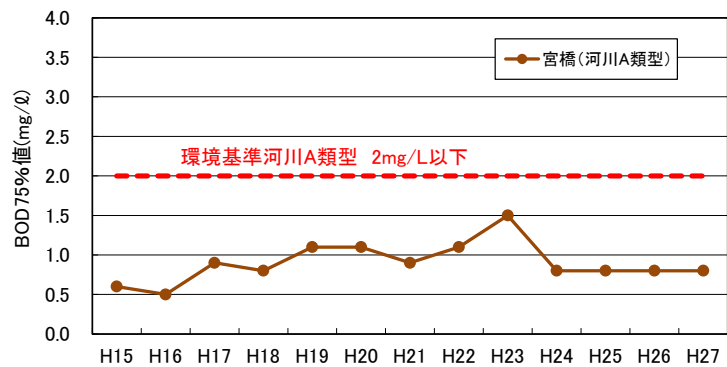
金剛川の主な地点における水質（BOD75%値）の経年変化状況
