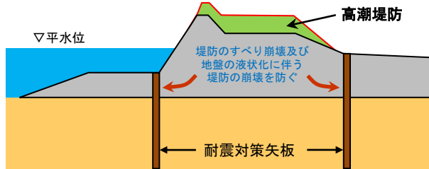
▲高潮・耐震対策イメージ
