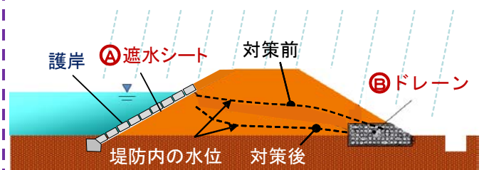
▲堤防補強(浸透対策)イメージ図
