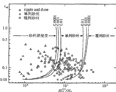
図 2-6.14 中規模河床形態の発生水理条件 20) (B: 川幅, H_0 : 河床勾配, H_0 : 水深, \tau_{*0} : 無次元掃流力)
