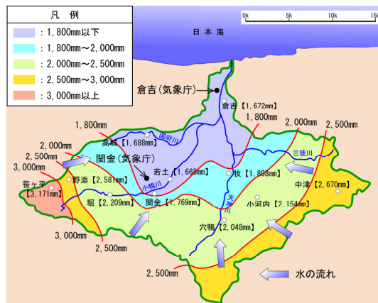
図 1.1.5 天神川流域の年間降雨量の分布 (H7~H16 年平均値)
