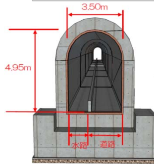
アーチカルバート 完成予想図
