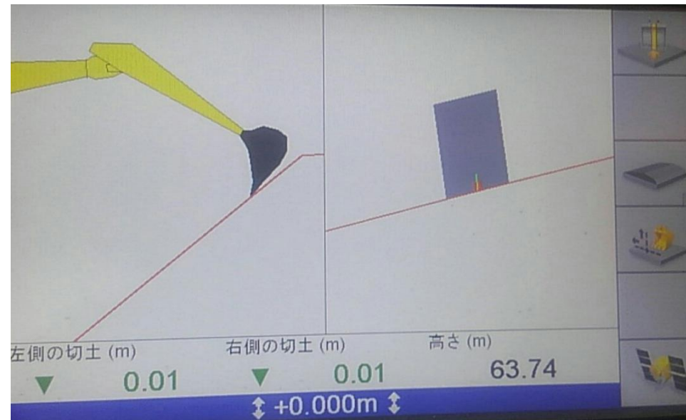
バックホウ運転席モニターを用いた法面整形
