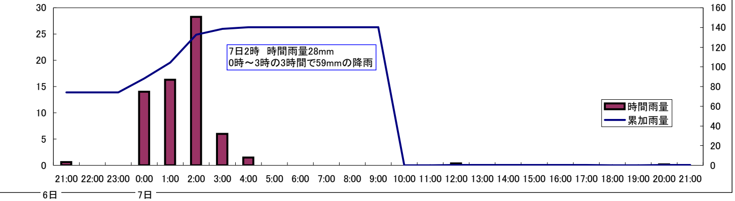
図-1 灰塚ダムの上流域で降った降雨の状況(流域平均雨量) (時間雨量:mm)
