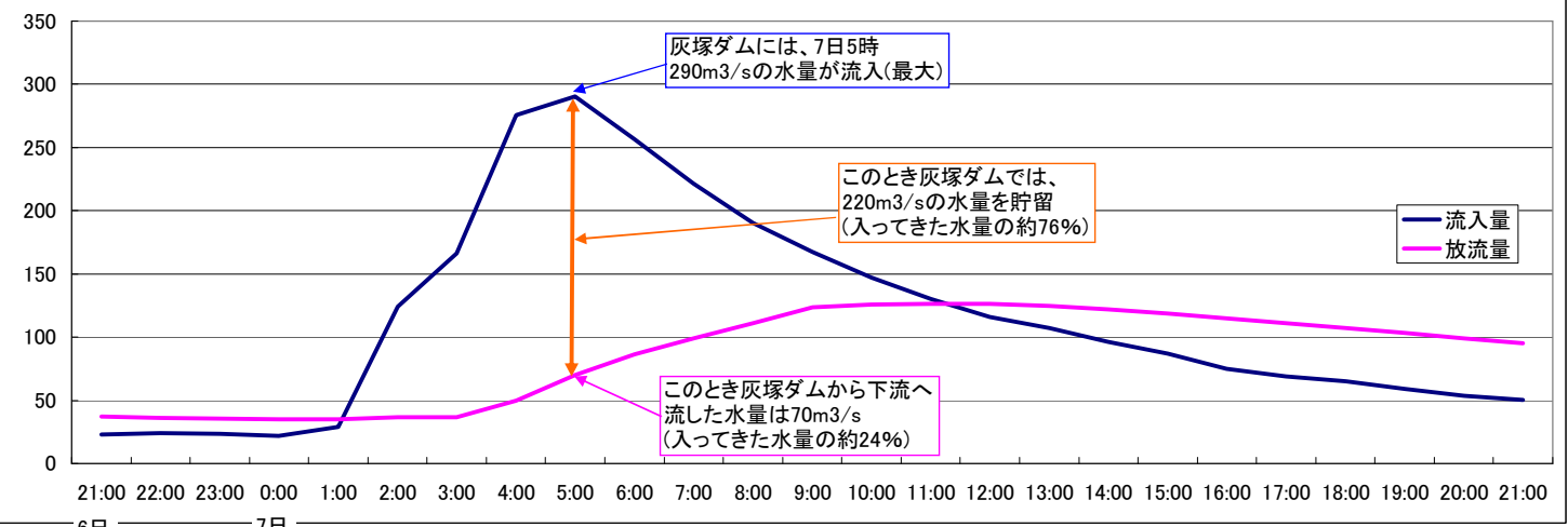
図-2 灰塚ダムへ流れ込んだ水量(流入量)とダムから下流へ流した水量(放流量)の状況
