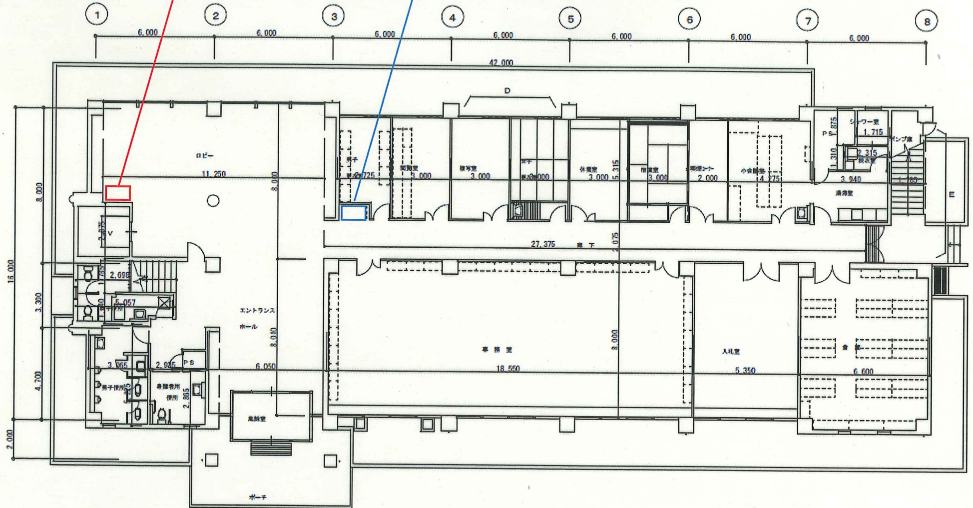
1階平面図
