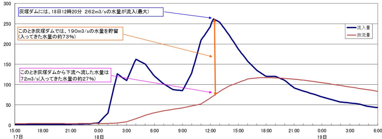
図-2 灰塚ダムへ流れ込んだ水量(流入量)とダムから下流へ流した水量(放流量)の状況
