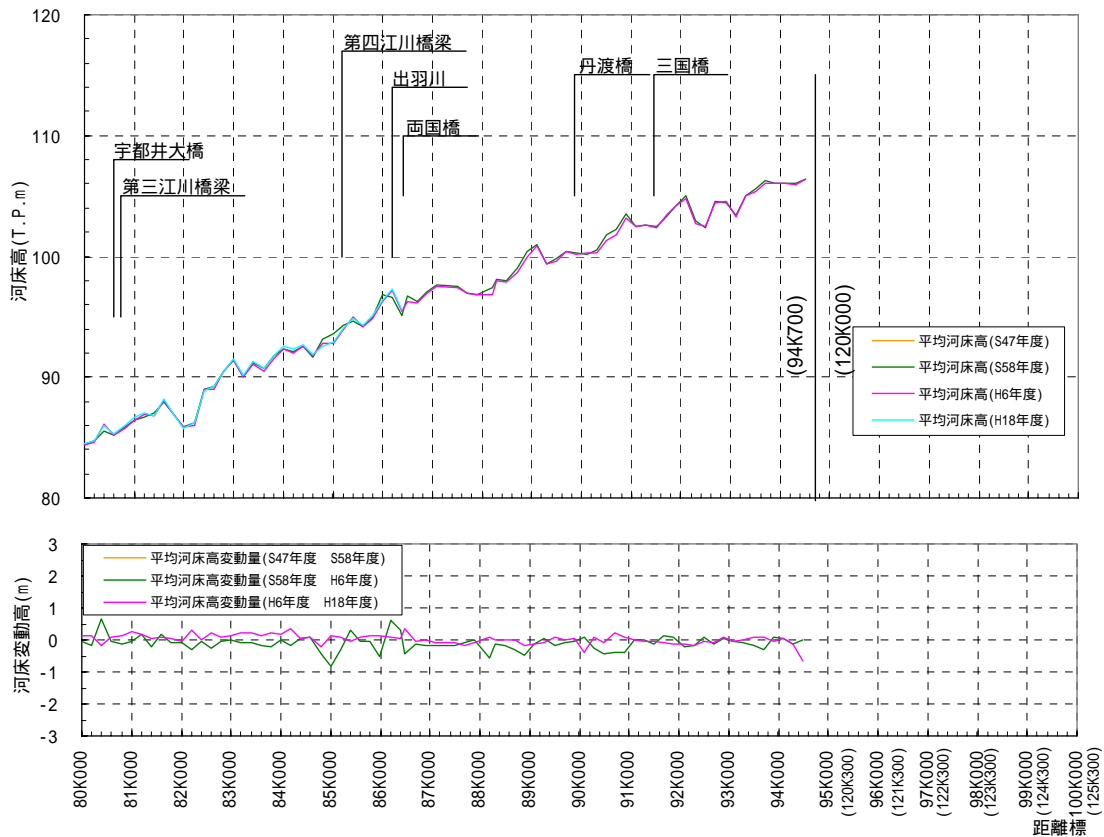
図 2-1(5) 低水路平均河床高縦断図(上)、河床変動縦断図(下)(江の川：80K000～100K000)
