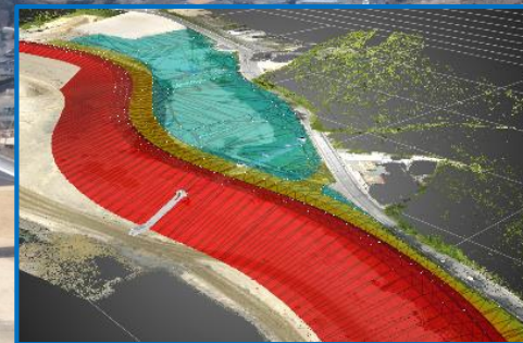
3次元設計データによる施工
