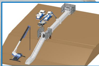
3Dモデルによる施工管理
