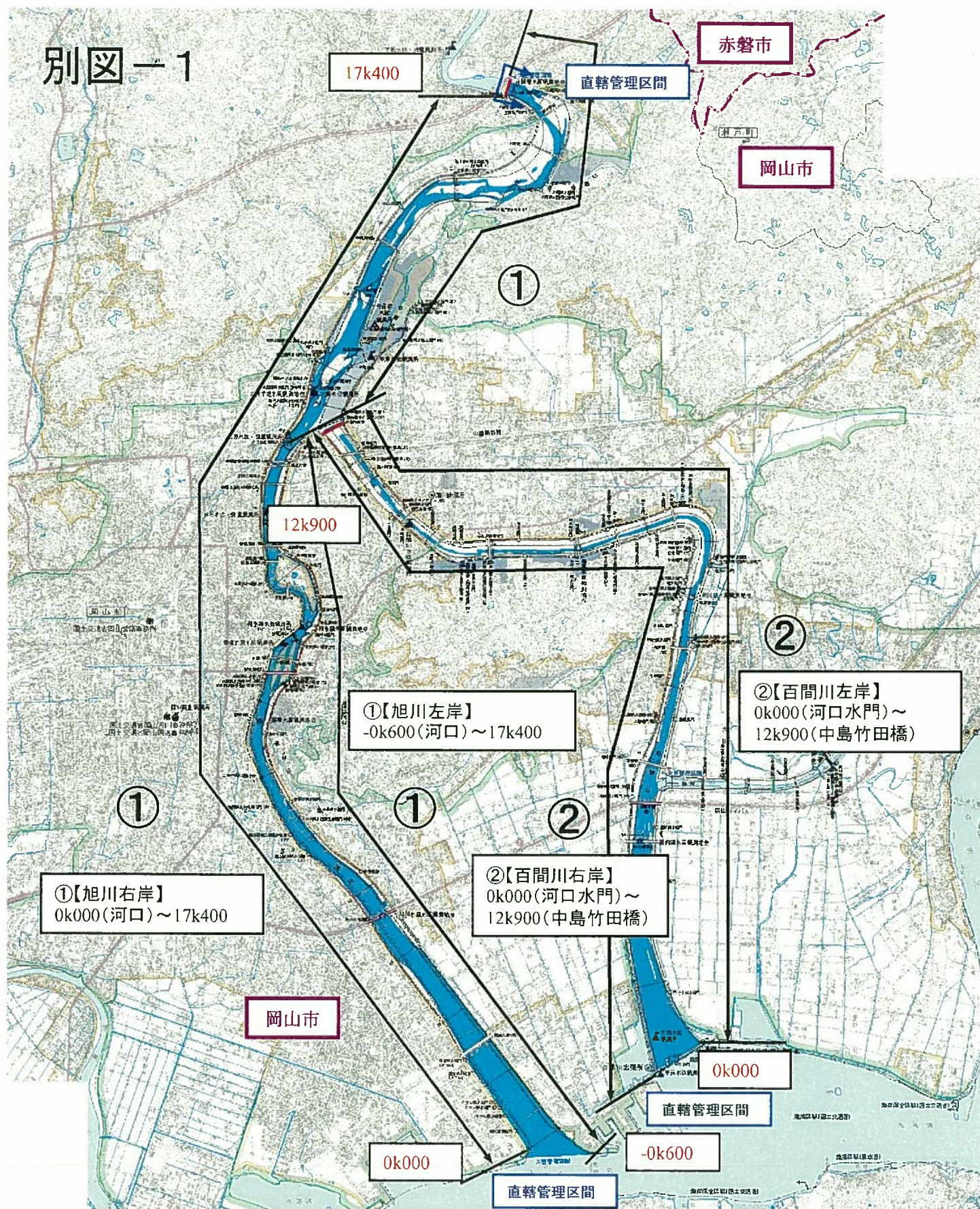
①災害応急対策活動等(測量・設計) 担当区間図(旭川)
