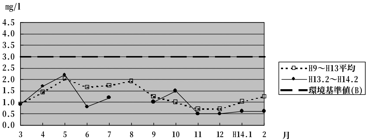
図－1 吉井川 永安橋の水質(BOD)
