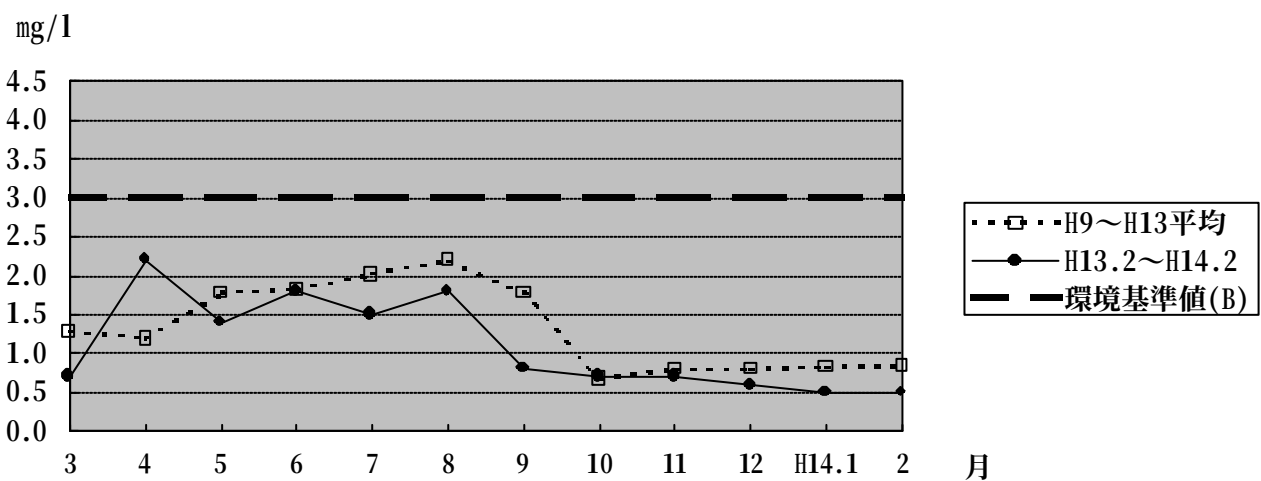
図－3 高梁川 霞橋の水質(BOD)
