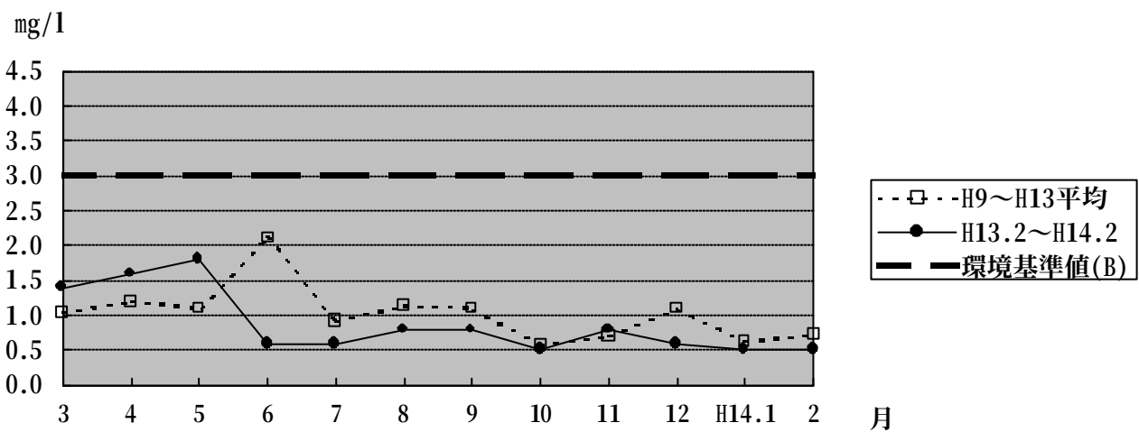
図－2 旭川 桜橋の水質(BOD)
