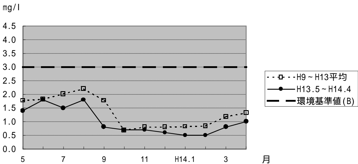
図 - 3 高梁川 霞橋の水質(BOD)
