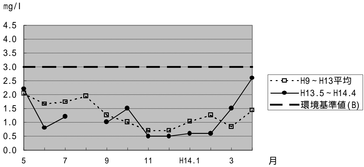
図 - 1 吉井川 永安橋の水質(BOD)
