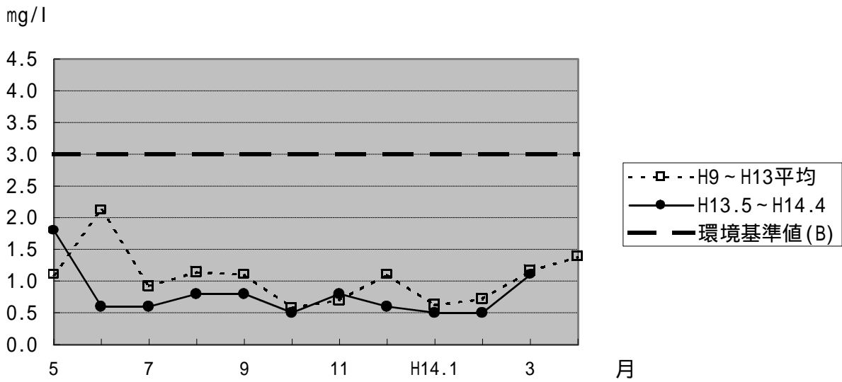
図 - 2 旭川 桜橋の水質(BOD)
