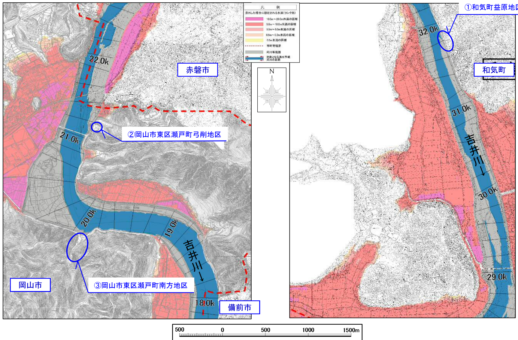
吉井川水系吉井川洪水浸水想定区域図（想定最大規模降雨）（平成29年4月19日公表） 抜粋
