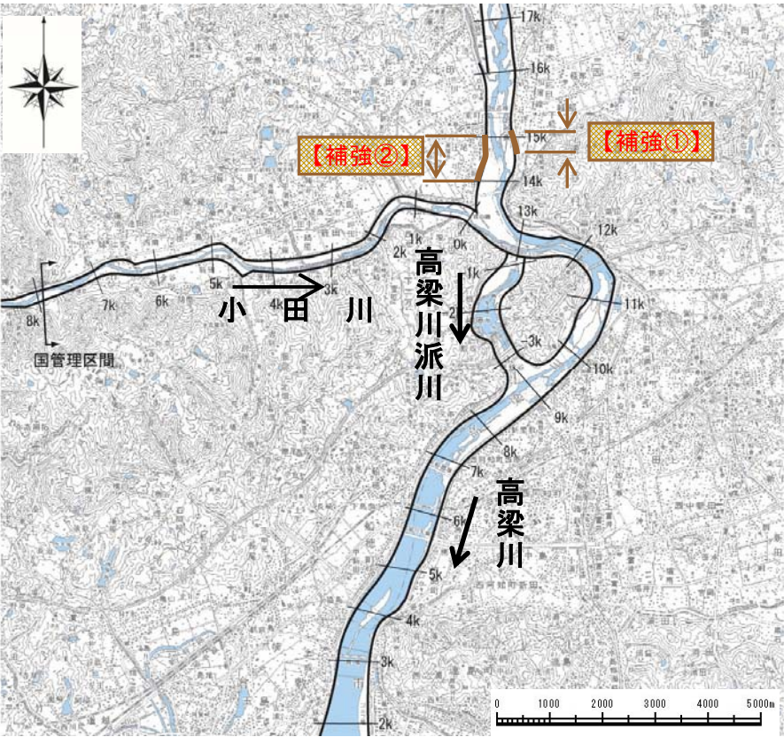
図 5. 1. 31 河川の整備を実施する区間の位置図（堤防構造を工夫する対策）
