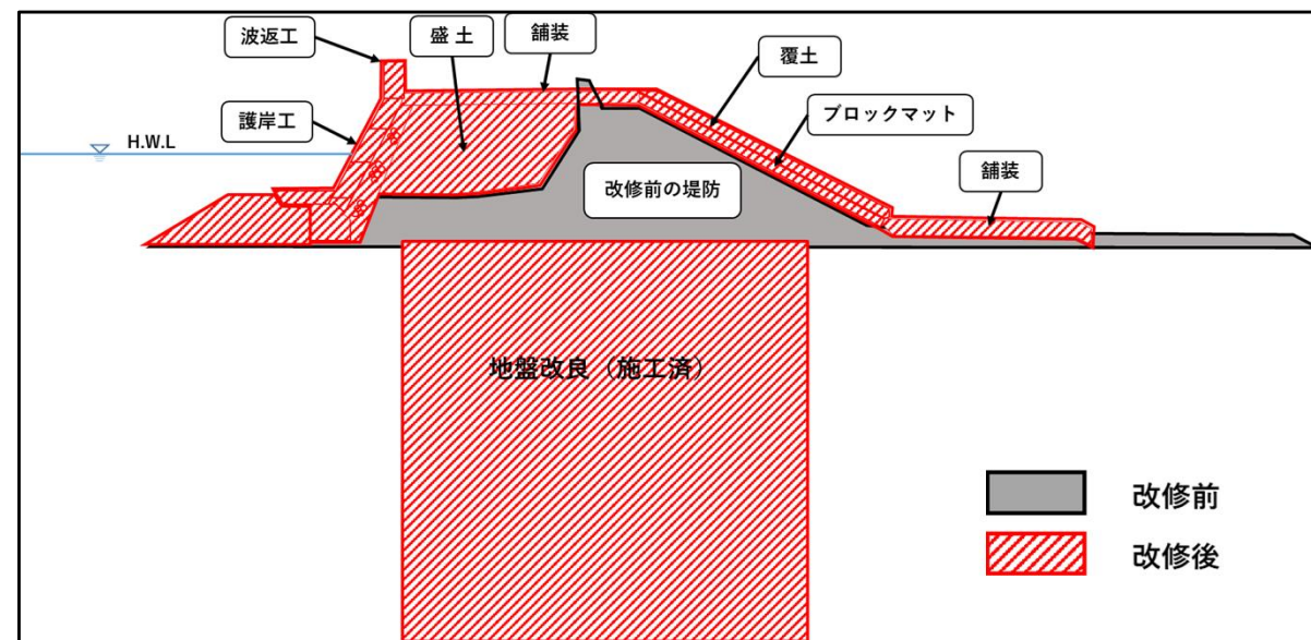
九幡地区 整備断面のイメージ図
