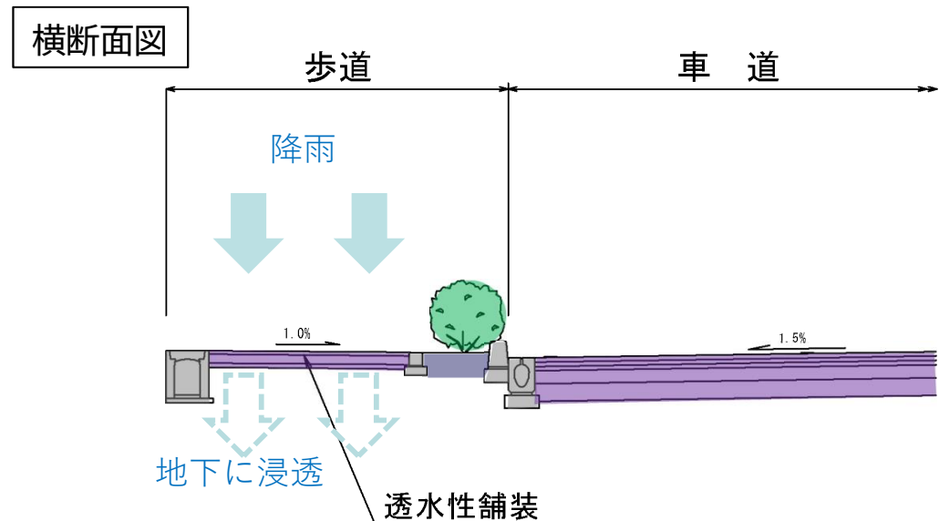
透水性舗装構成図
