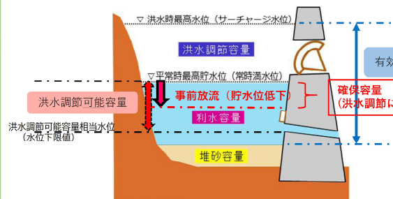
多目的ダム(ゲート有り) 吉田ダム・八塔寺川ダム等
