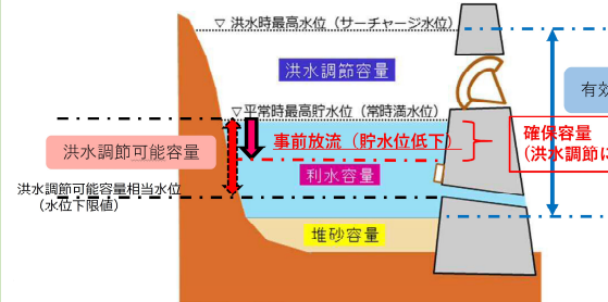
多目的ダム(ゲート有り) 湯原ダム・旭川ダム等
