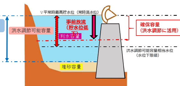
利水ダム 山手ダム・北房ダム・社口ダム等
