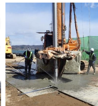
耐震対策の施工状況 (九幡地区)
