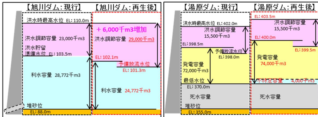
貯水池容量配分図
