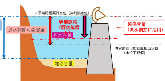
利水ダム 恩原ダム等
