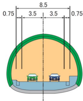
《トンネル断面図》
