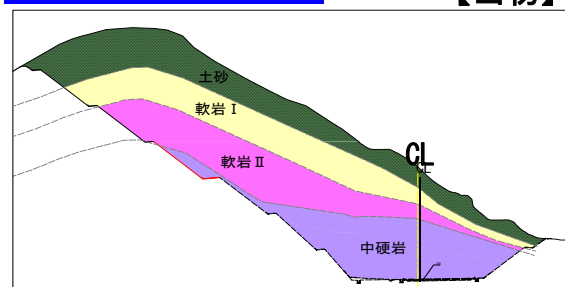
横断 (A-A断面)
