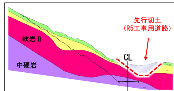
横断 (A-A断面)
