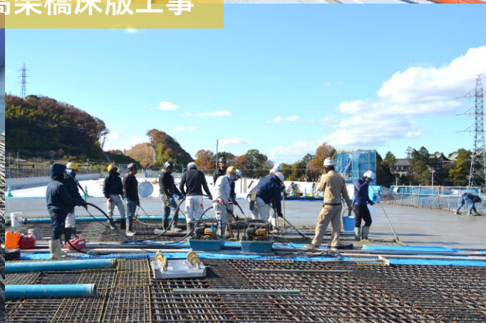
入江高架橋床版工事
