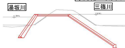
導流堤の改良イメージ
