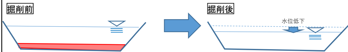
河道掘削による水位低下のイメージ
