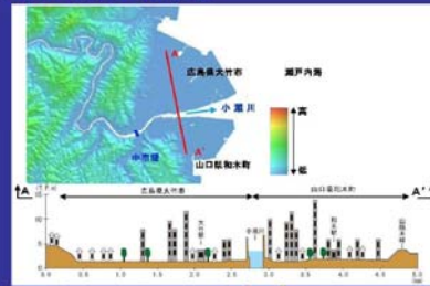
小瀬川河口地区を中心とした地盤高図と河口地区の横断面図
