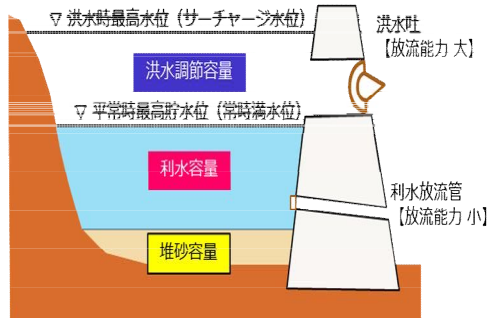
ダム容量の内訳
