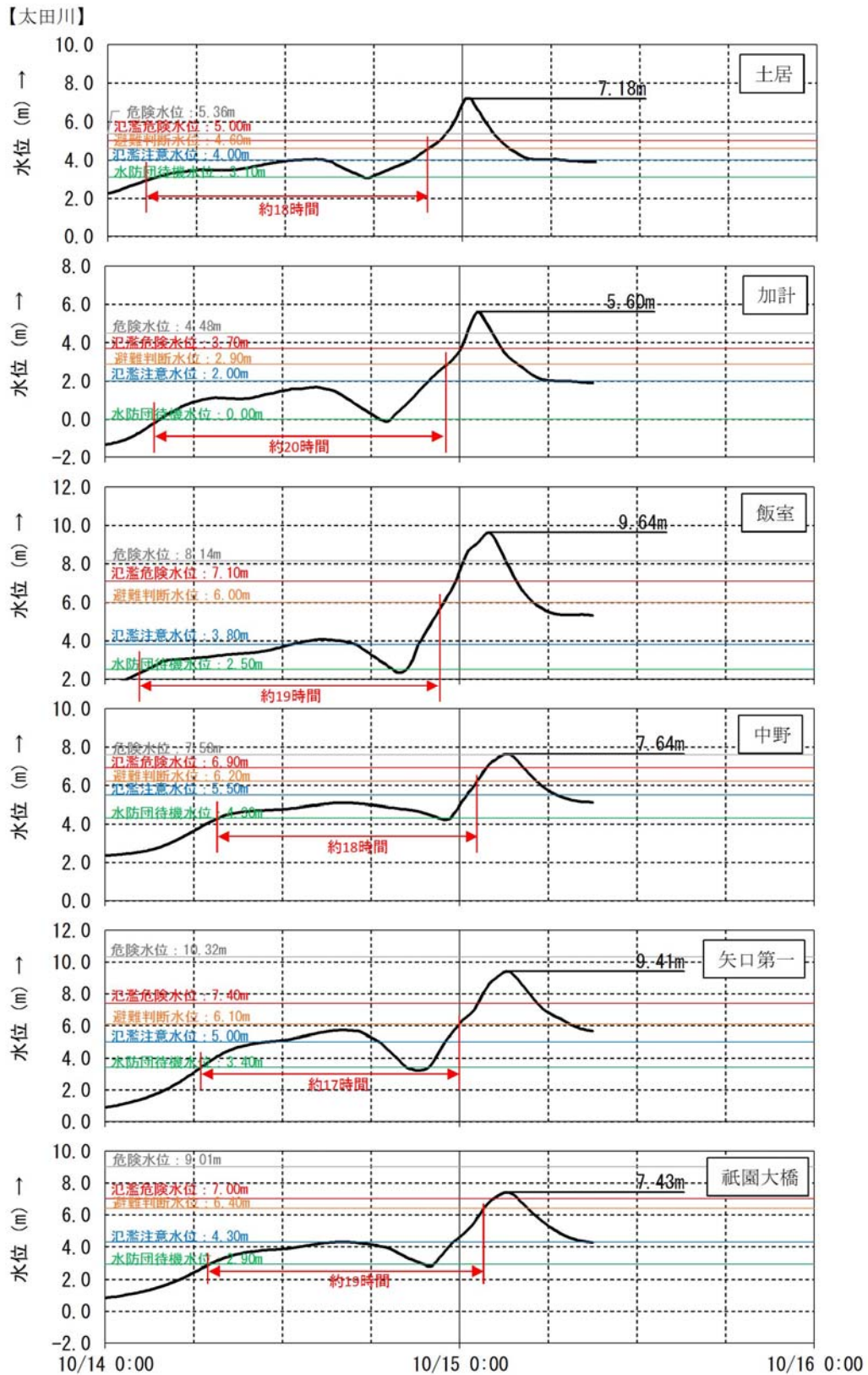
図 4-2 (1) 想定する水位波形
