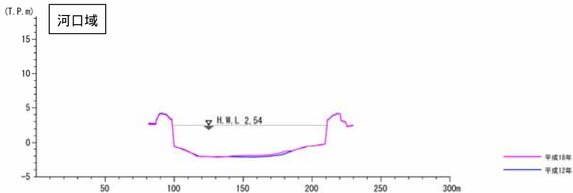
図 経年变化横断面図(市内派川：京橋川)
