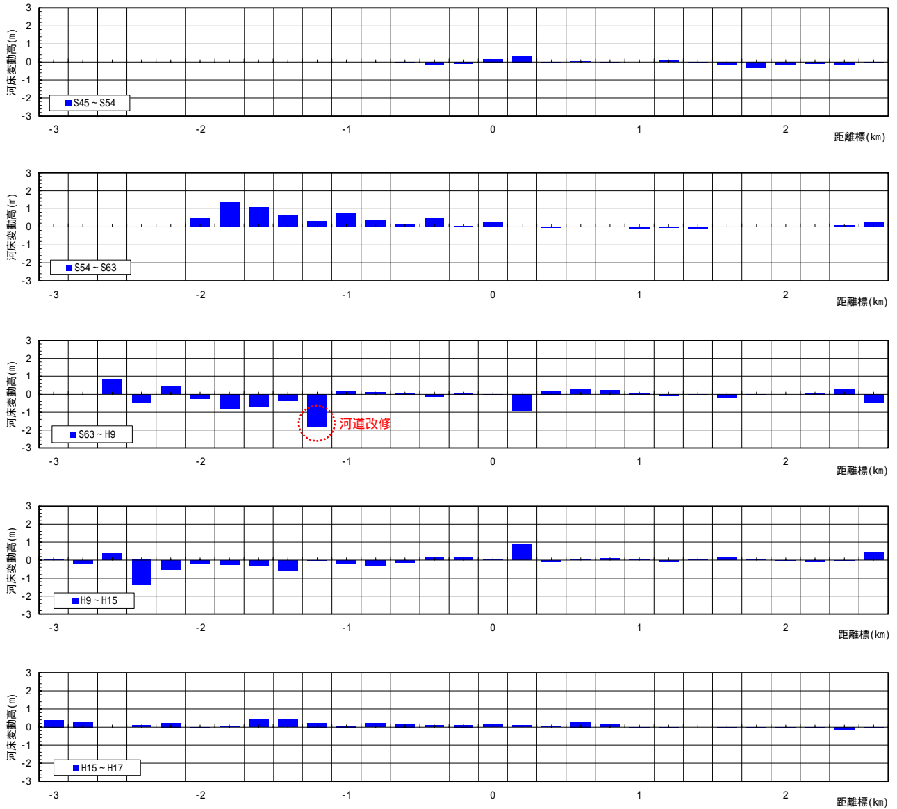
圖 2-8(3) 低水路内河床變動量經年变化図(市内派川：元安川)
