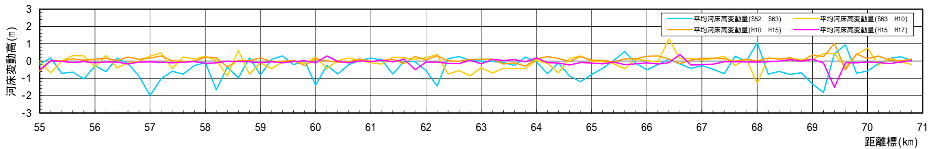
図 2-2(5) 河床変動縦断図(太田川本川 : 55K000 ~ 70K800)
