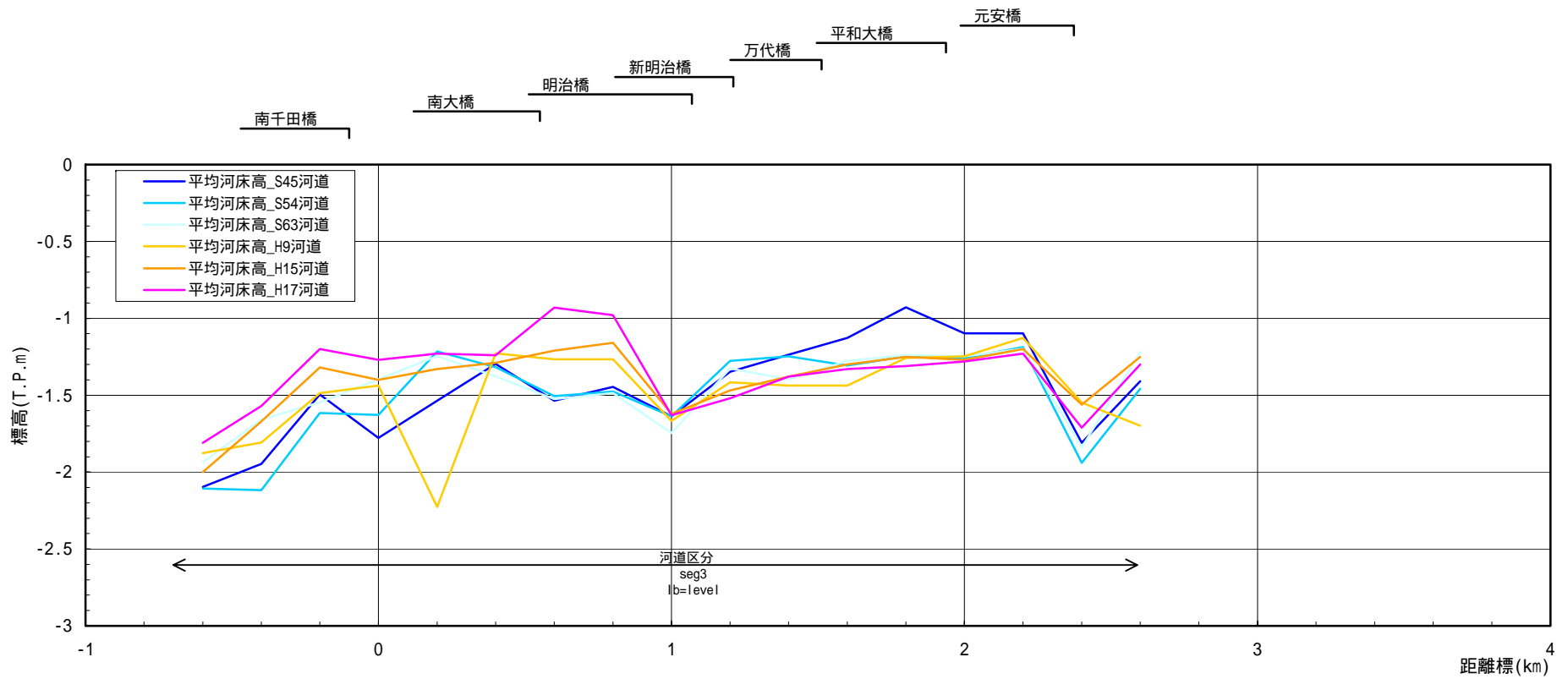
图 2-3(3) 低水路平均河床高縦断図(市内派川：元安川)
