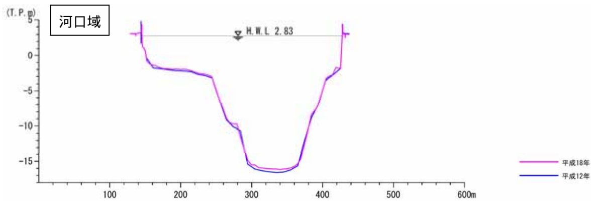
図 経年变化横断面図(市内派川：猿猴川)
