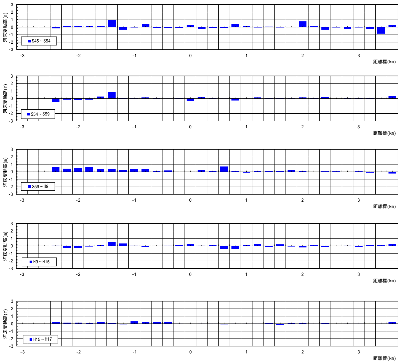
図 2-8(1) 低水路内河床變動量経年变化図(市内派川：天満川)
