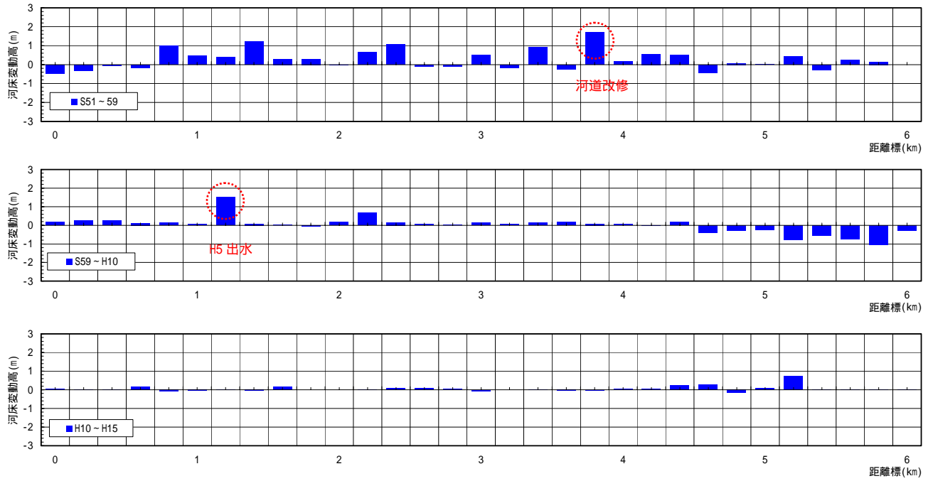
图 2-9(1) 低水路内河床变动量经年变化图(支川：第 1 古川)
