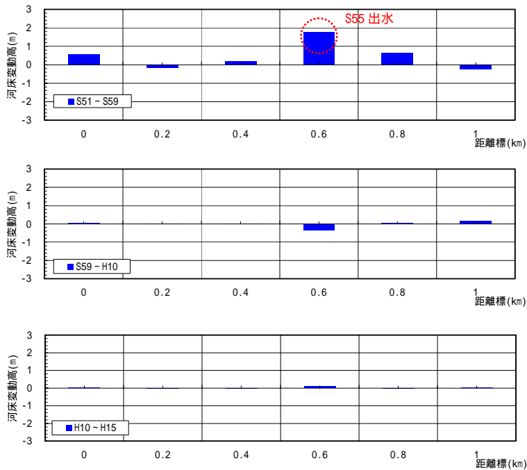
图 2-9(2) 低水路内河床变动量经年变化图(支川：第 2 古川)
