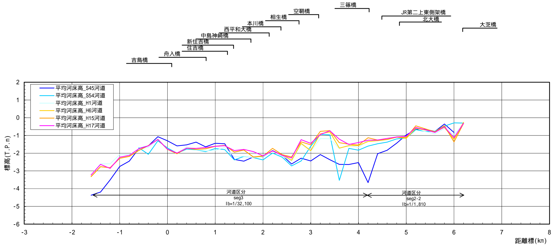
図 2-3(2) 低水路平均河床高縦断面図(市内派川：旧太田川)
