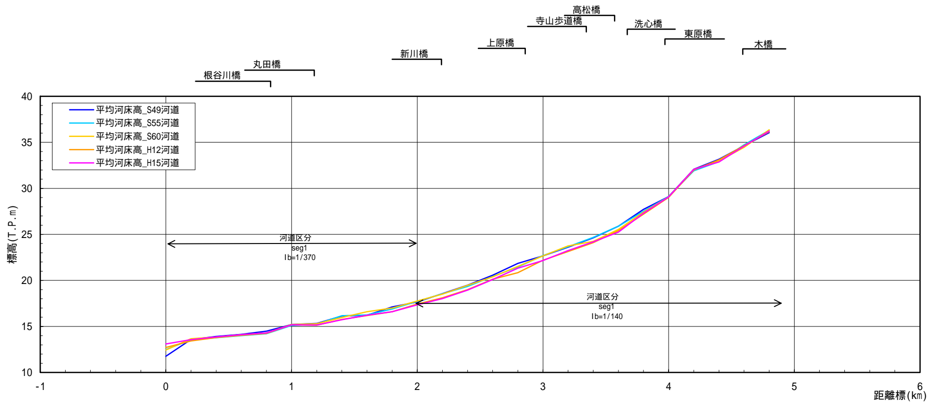
図 2-5(4) 低水路平均河床高縦断図(支川：根谷川)
