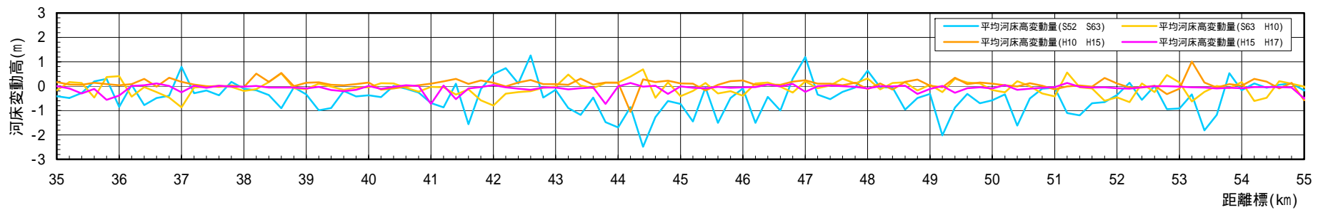
図 2-2(4) 河床変動縦断面図(太田川本川：35K000～55K000)
