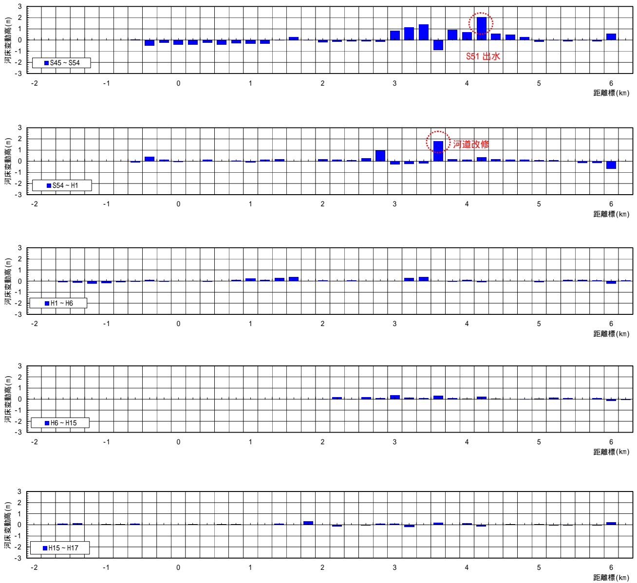
図 2-8(2) 低水路内河床變動量経年变化図(市内派川：旧太田川)
