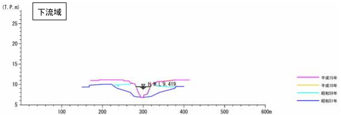
図 2-12(2) 経年变化横断面図(支川：第2古川)
