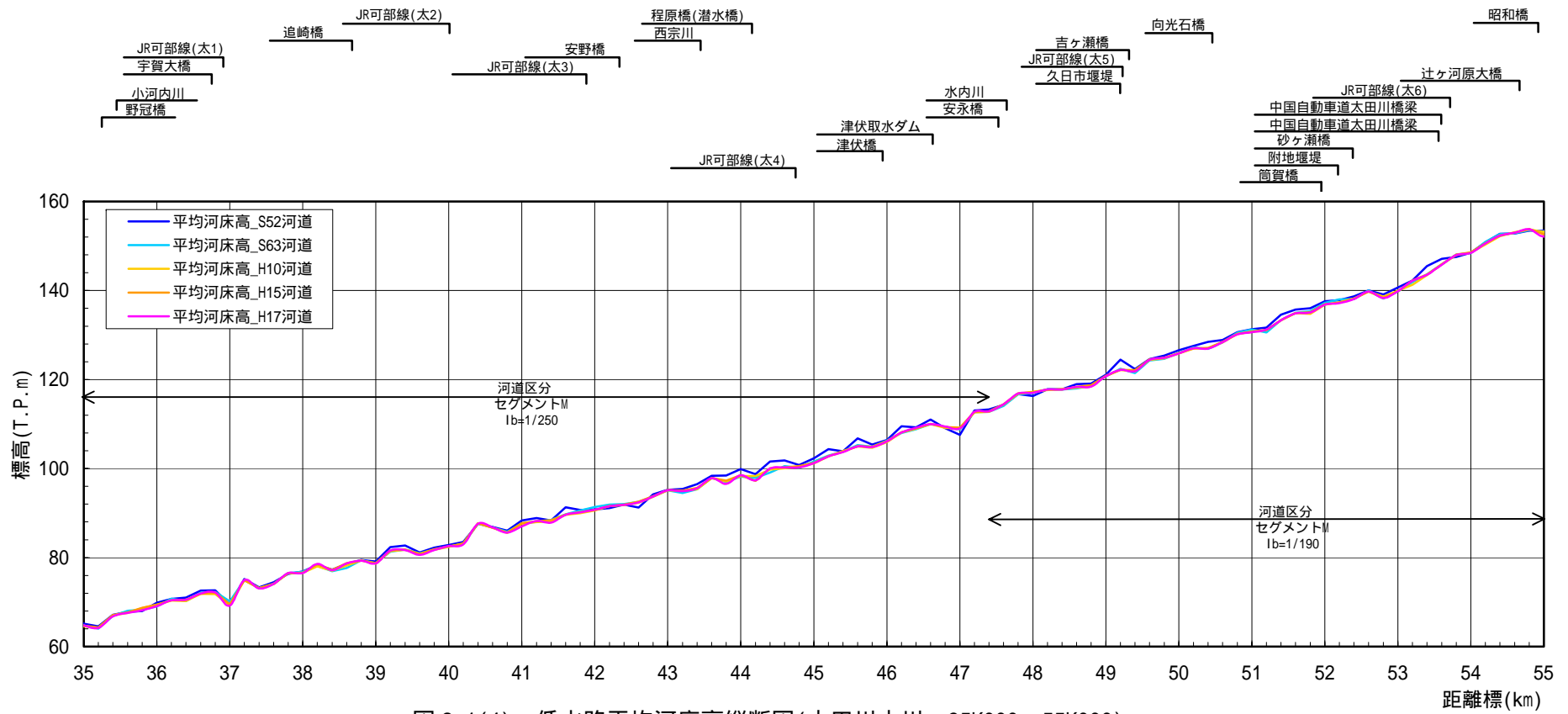
図 2-1(4) 低水路平均河床高縦断面図(太田川本川：35K000～55K000)
