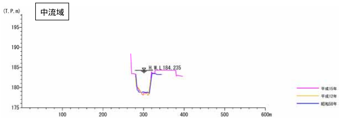
図 2-12(6) 経年变化横断面図(支川：中祖川)
