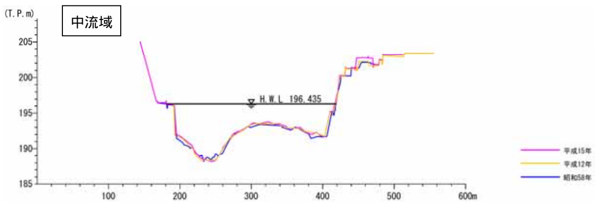
図 2-12(5) 経年变化横断面図(支川：滝山川)
