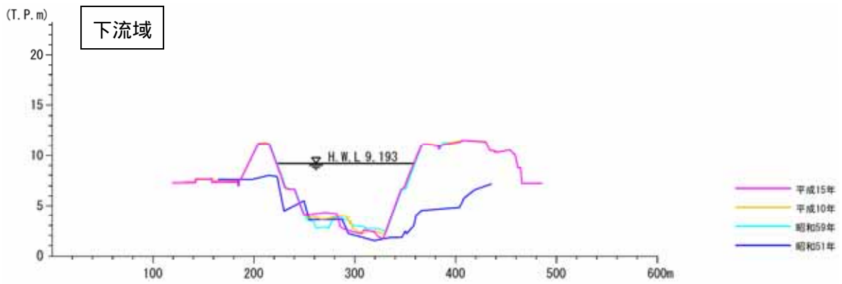
図 2-12(1) 経年变化横断面図(支川：第1古川)
