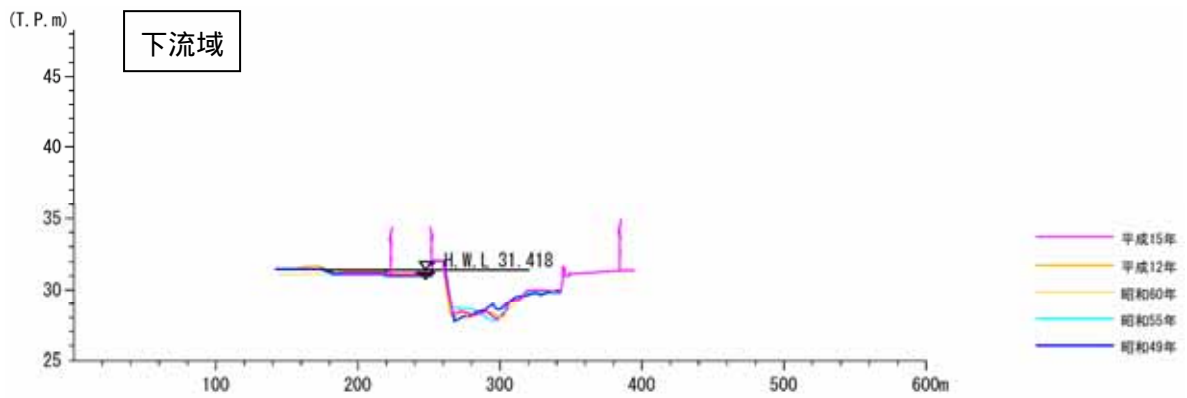
図 2-12(4) 経年变化横断面図(支川：根谷川)
