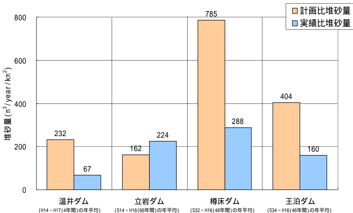
図 3-1 ダム堆砂量
