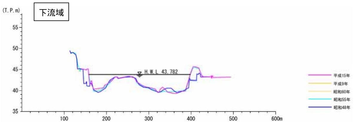
図 2-12(3) 経年变化横断面図(支川：三篠川)
