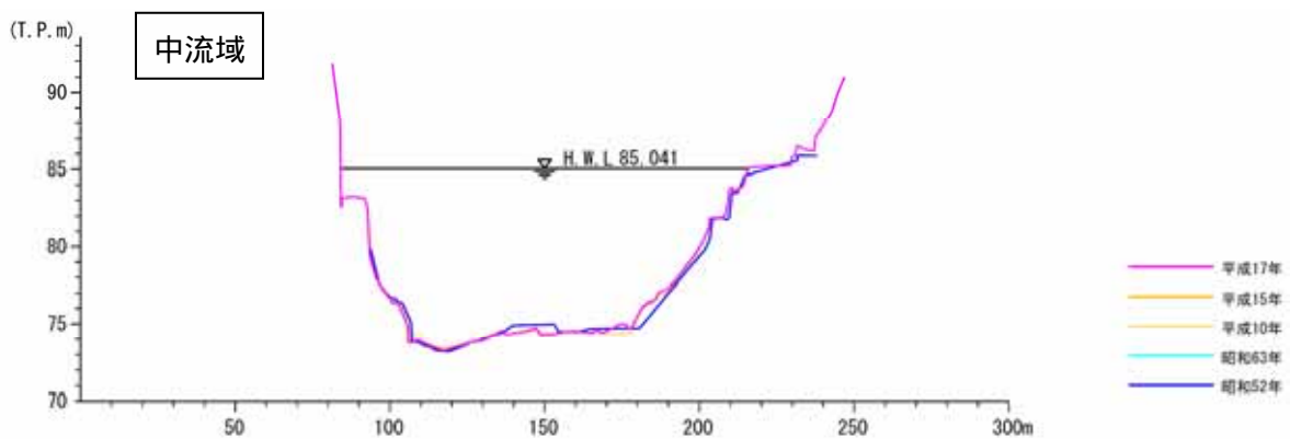
図 2-10 経年变化横断面図(太田川本川)
