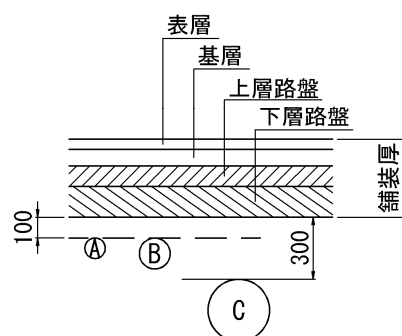
車道部（交通量多）
