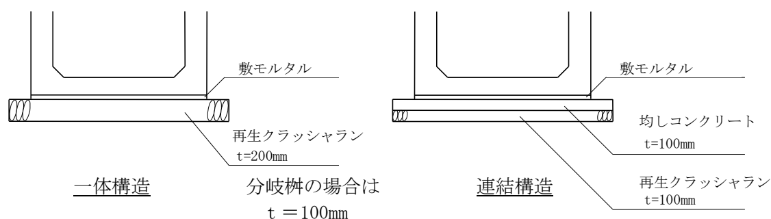
図 3-6-2 特殊部の基礎構造
