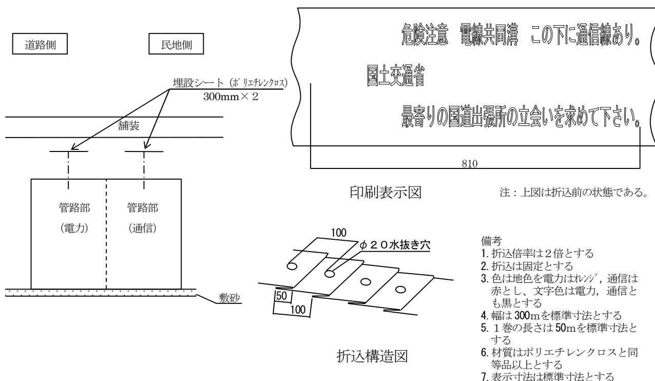
図3-2-1 埋設シートによる保安対策
