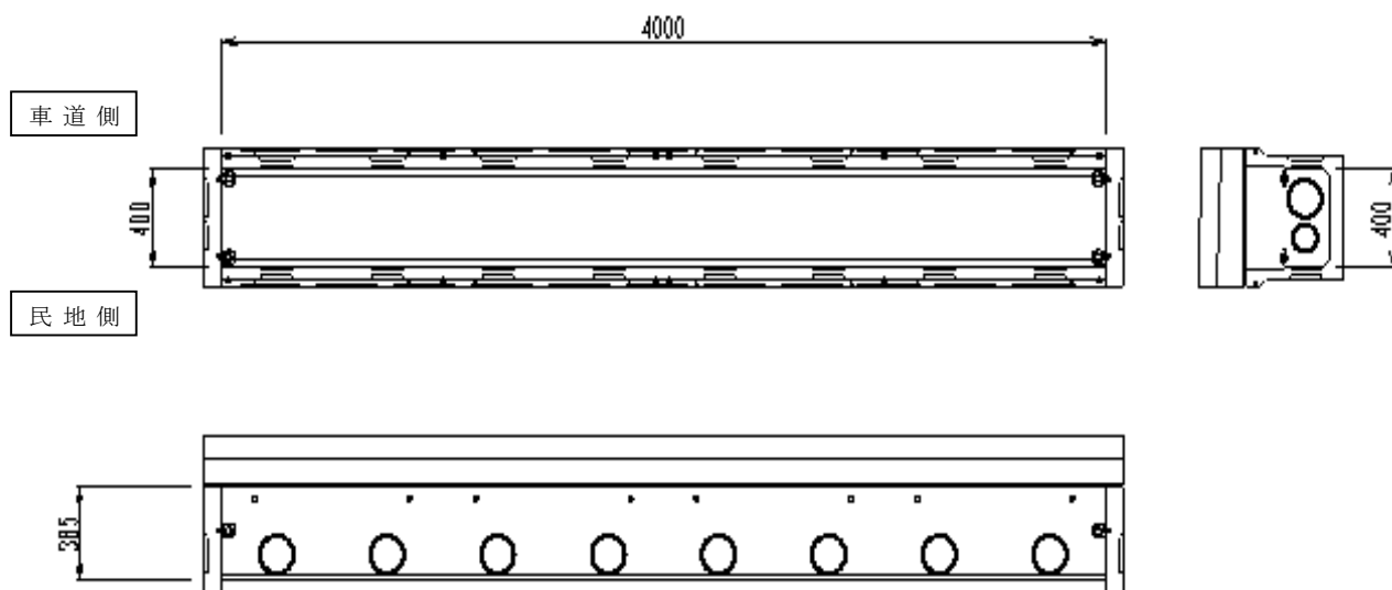
図 3-5-2 簡易トラフ概略構造図
