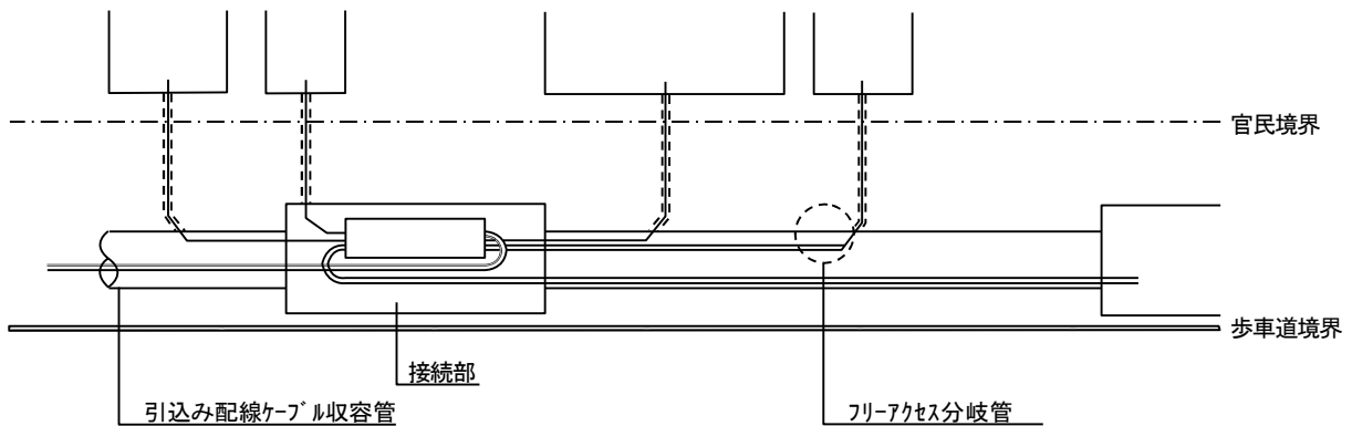
図 1-2-4 概略平面図
