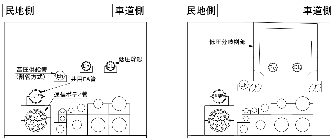
図 1-3-1 浅層埋設方式標準断面（一般部、低圧分岐桝部）
