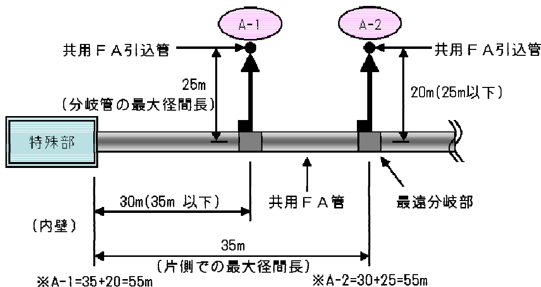
図 3-1-8 共用F A引込み管長
