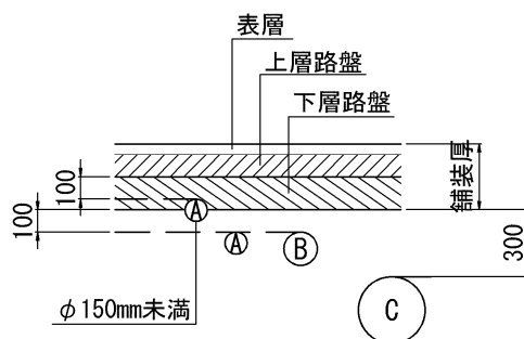
車道部（交通量少）
