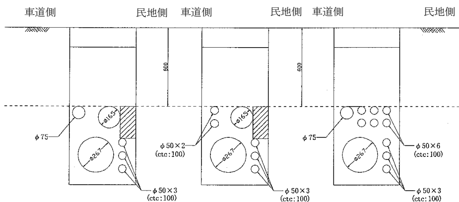
図 3-4-3 連系管・引込管の通信接続枳端壁部取付例（ボディ管φ250）
