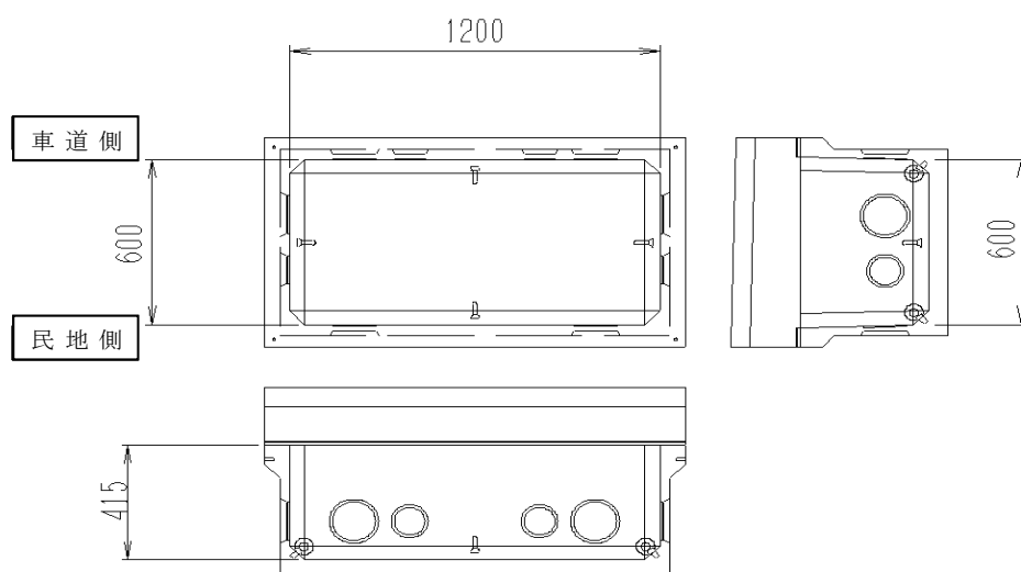
電力Ⅱ型（2引込み用）
