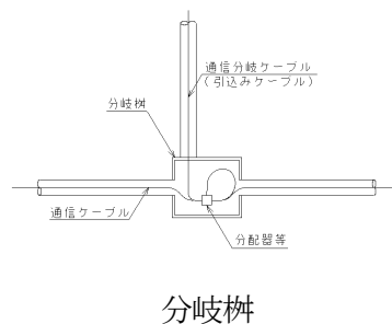
図 1-2-3 通信分岐構造概略図
