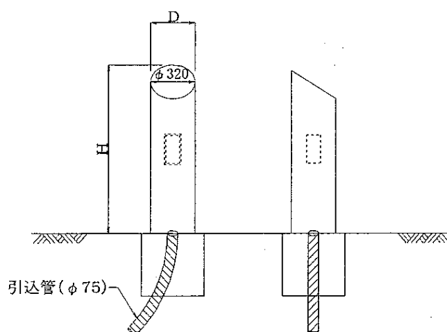
図 3-5-6 ペDESTALボックス IV型
