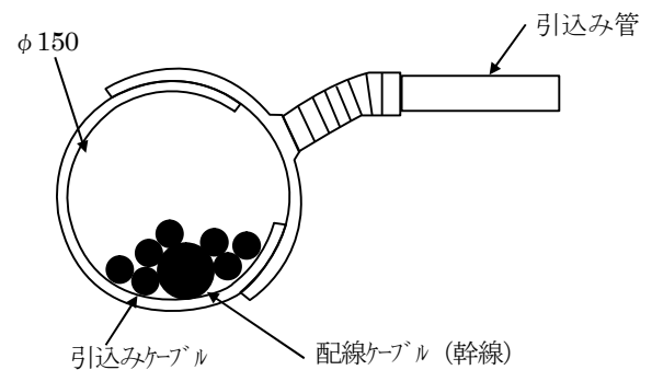
フリーアクセス分岐管断面図
