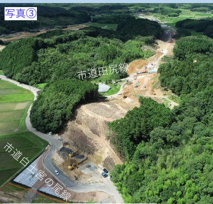
写真③ 金道地区第2改良工事 金道地区伐採作業 状況
