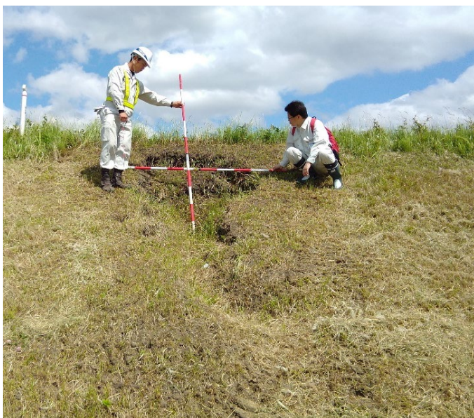
法面の崩れの状況(高梁川)
