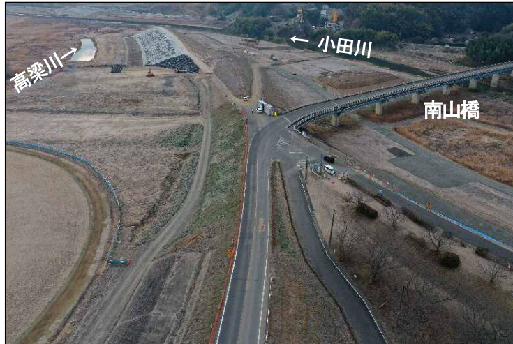
②小田川上流から見た上流締切堤防
