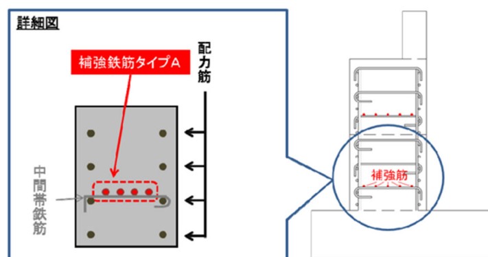
図 9-4-4 ひび割れ発生方向と抵抗鉄筋概要図 (補強鉄筋タイプ A)
