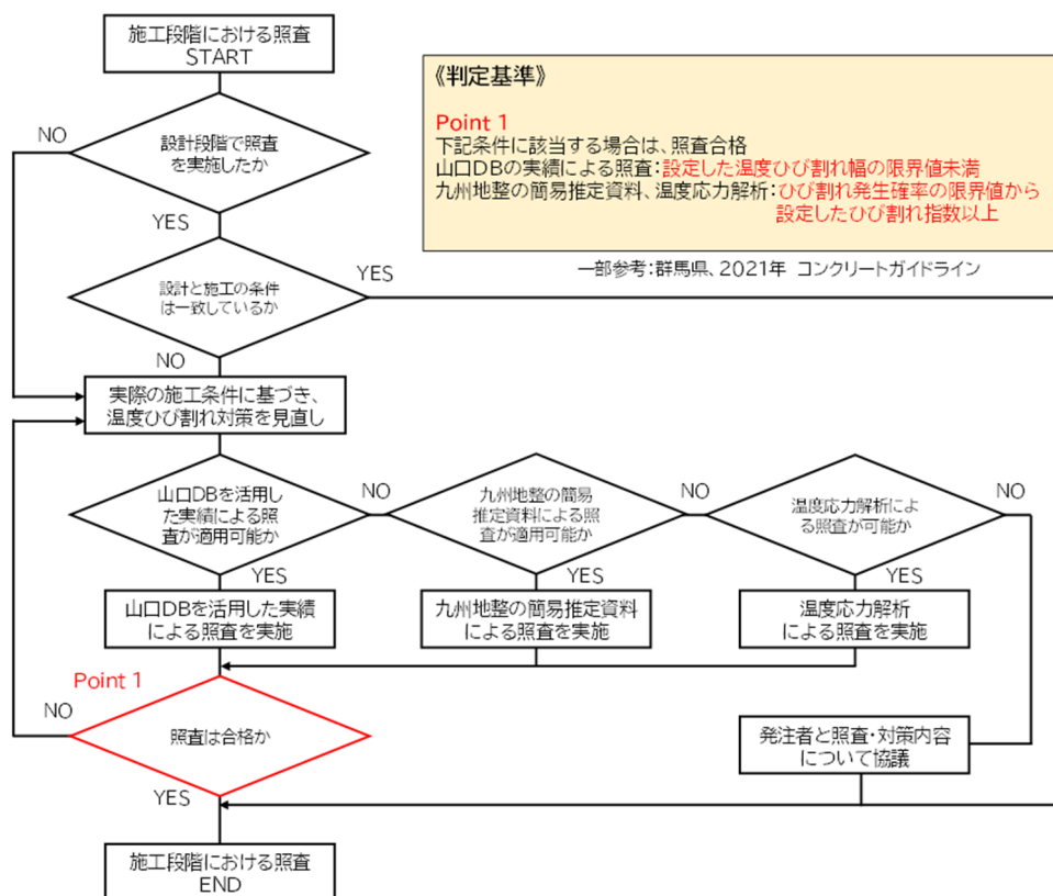
図9-6-3 施工段階における温度ひび割れの照査フロー
