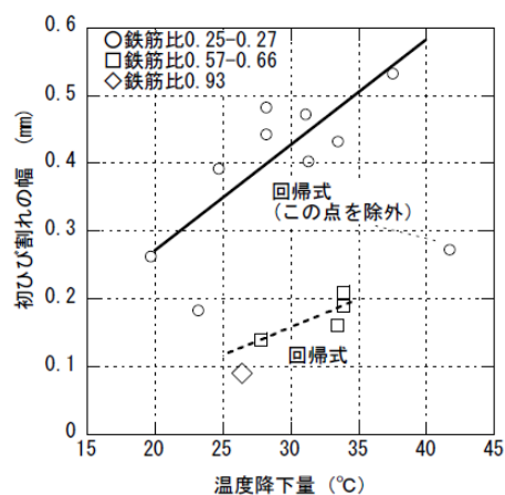
図9-2-11 温度降下量と温度ひび割れの幅の関係
