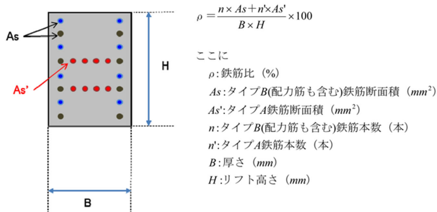
図9-4-7 補強鉄筋タイプA+B
