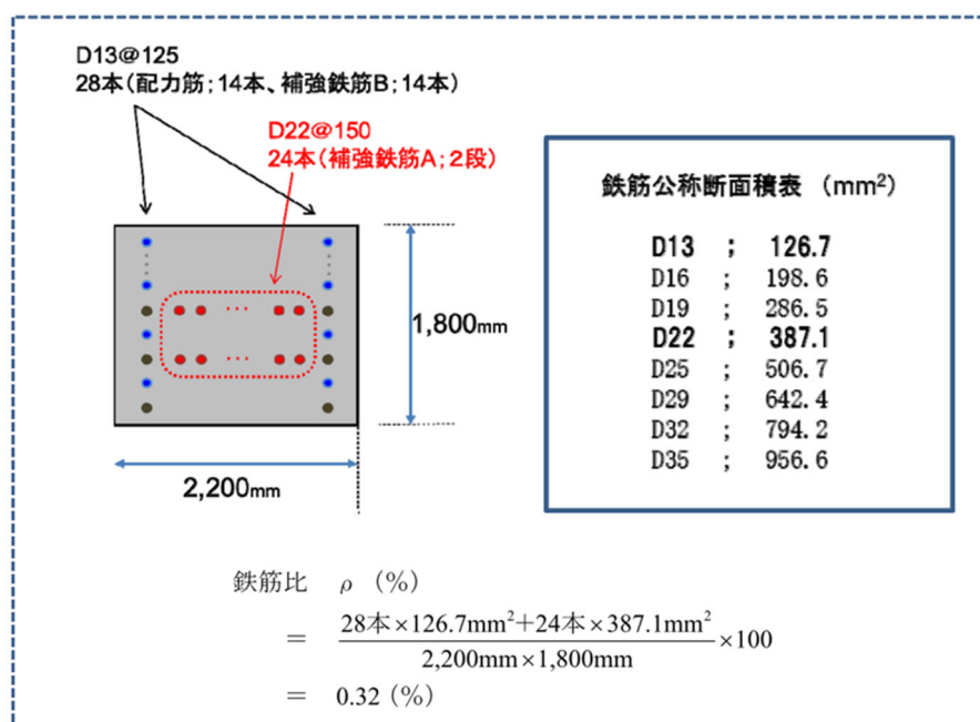
図9-4-8 鉄筋比の算出例
