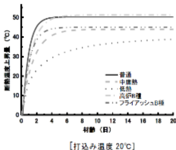
図9-2-5 各種セメントを用いたコンクリートの断熱温度上昇曲線
