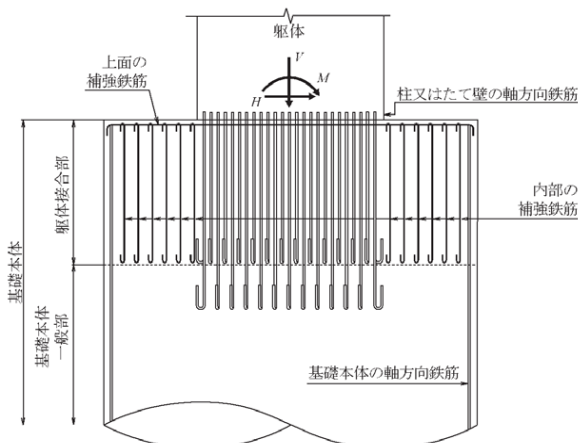
図 4-1-21 柱状体深礎基礎各部の構造例
