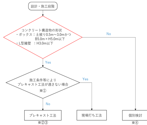
図3. 工法選定フロー
