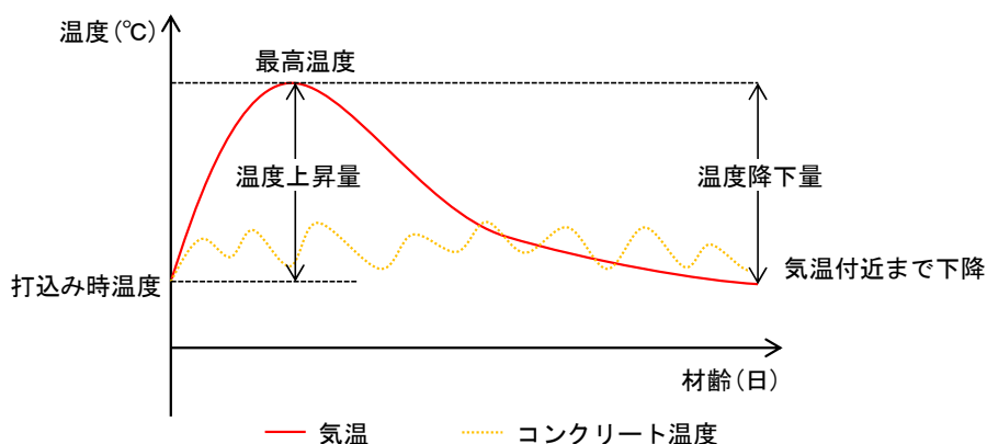
図9-2-2 コンクリート打込み後の温度変化
