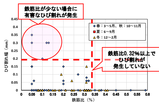
図9-2-12 鉄筋比と温度ひび割れ幅の関係
