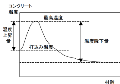
図9-2-6 マスコンクリートの温度変化
