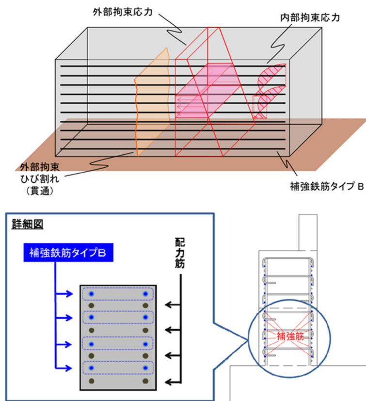
図 9 - 4 - 5 ひび割れ発生方向と抵抗鉄筋概要図 (補強鉄筋タイプ B)
