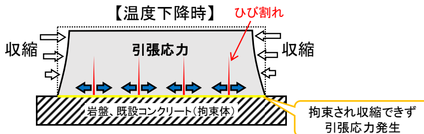
図 9-2-4 外部拘束による温度ひび割れ
