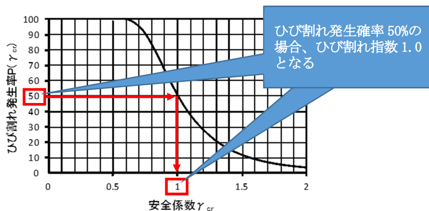
図 9-4-2 安全係数 \gamma_{cr} （ひび割れ指数 I_{cr}(t) ）とひび割れ発生確率（3次元解析の場合）
