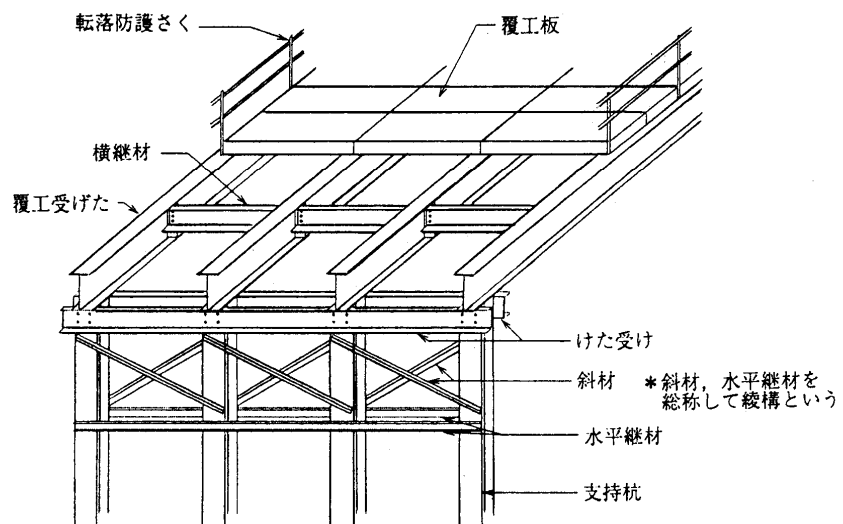
仮橋名称図
