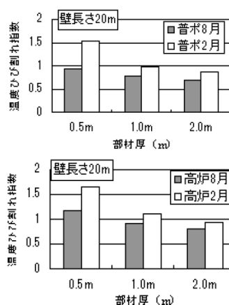
図9-2-7 施工時期による最高温度への影響
