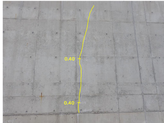
図9-2-1 温度ひび割れの例（前のリフトの外部拘束により発生）
