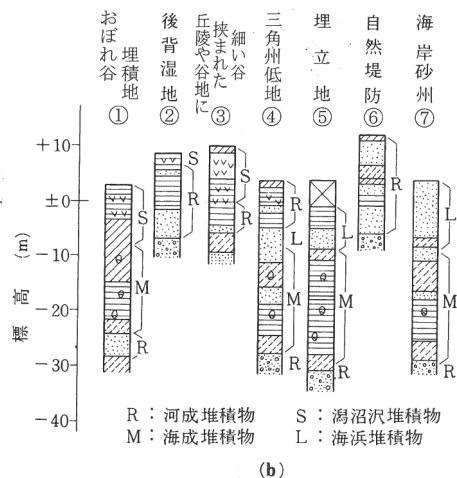
図 3-1-1 軟弱地盤の分布と成層例
