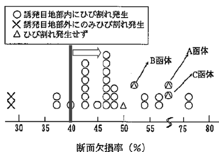
図9-2-9 断面欠損率と温度ひび割れ の関係
