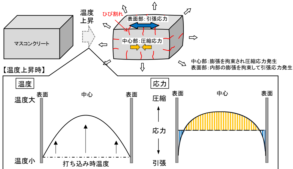
図 9-2-3 内部拘束による温度ひび割れ
