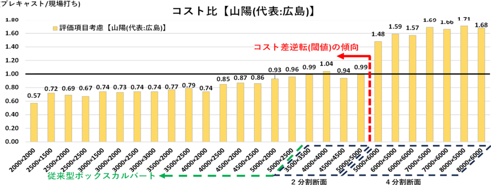
図1. 経済比較結果 (ボックスカルバート)
