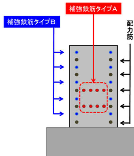
図 9 - 4 - 6 補強鉄筋タイプ A+B
