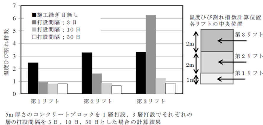
図9-2-8 温度ひび割れ指数に及ぼす打継ぎ間隔の影響
