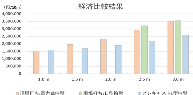
図2. 経済比較結果 (L型擁壁)
