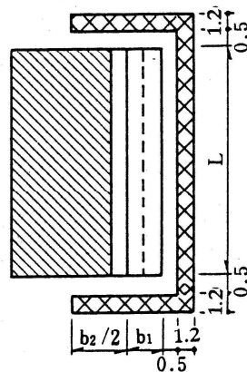
③ 平面図
