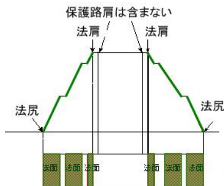
《作図例》
