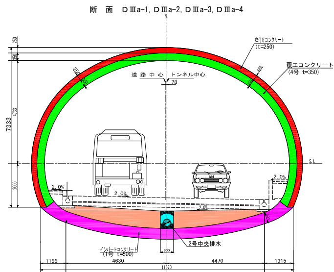
標準断面図
