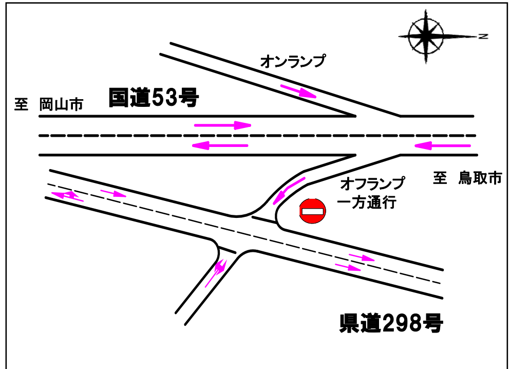
改良後交差点
