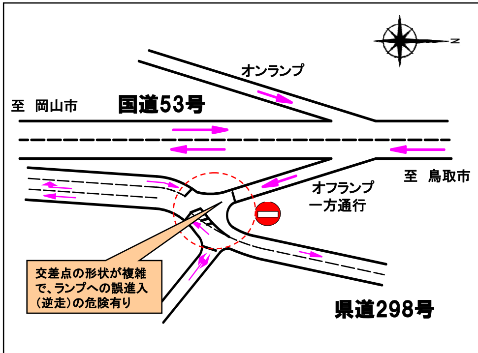
改良前交差点
