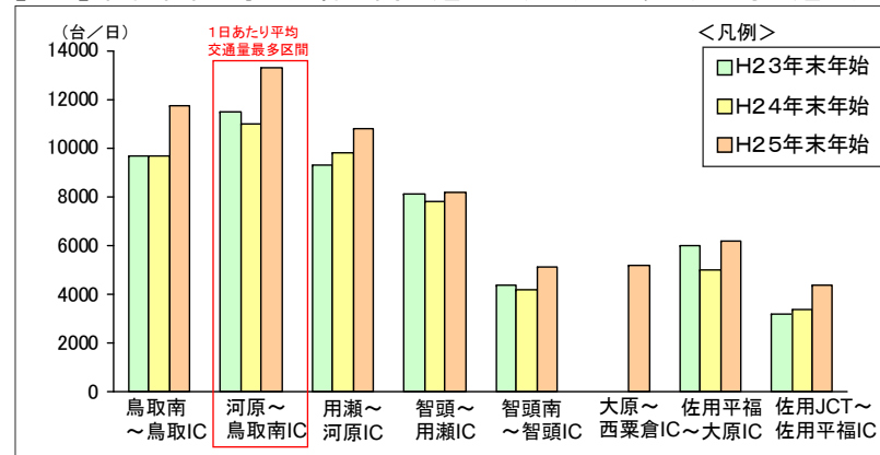
【図1】年末年始 鳥取道各IC間交通量グラフ(1日あたり平均交通量)
