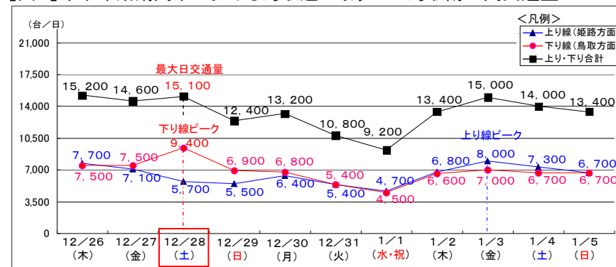
【図2】年末年始期間中における鳥取道 河原IC～鳥取南IC間交通量
