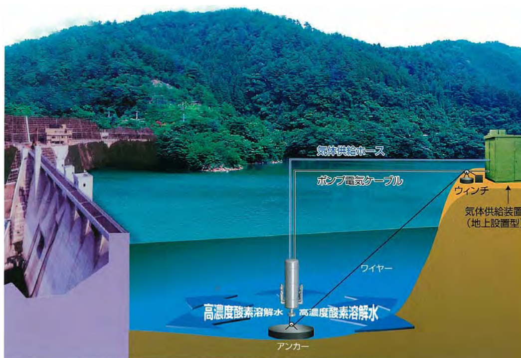
図 3-1 高濃度酸素溶解装置（湖底アンカー式）概念図
