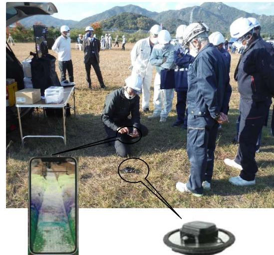
(3次元測量表示例) (GNSSレシーバー) スマホで測量対象物をスキャンする だけ、誰でも簡単3次元測量
