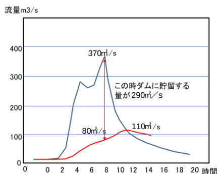
島地川ダム洪水調節計画図
