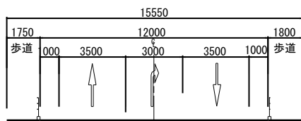
工事前断面図
