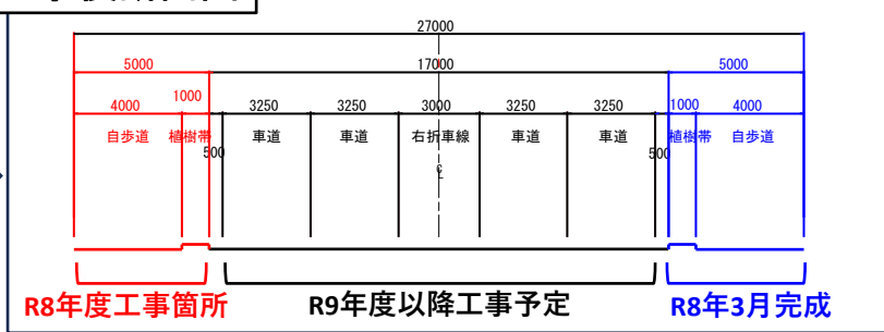
工事後断面図
