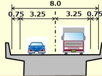
<橋梁部>
