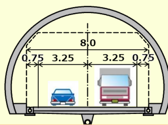
<トンネル部>
