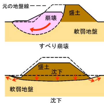
軟弱地盤による崩壊メカニズムの例
