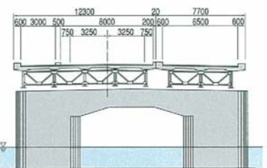
橋梁断面図
