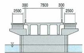
橋梁断面図
